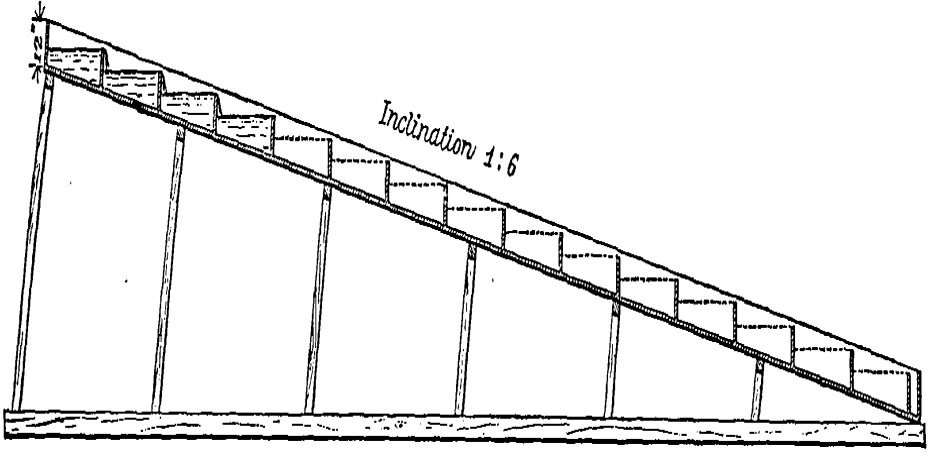
Longitudinal Section
